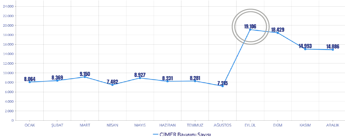
Grafik 2: 2025 Yılı Aylara Göre Başvuru Dağılımı
